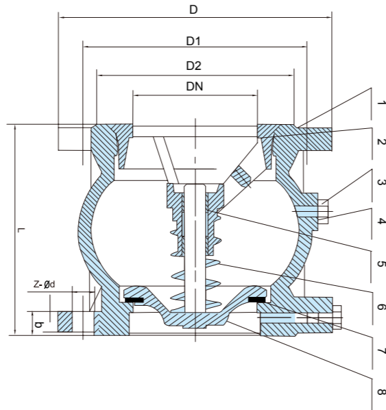
DIN Cast Iron Silent Check Valve PN16
